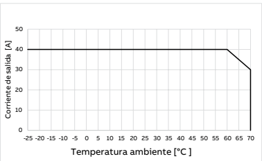
CP-S.1 24/40.0
