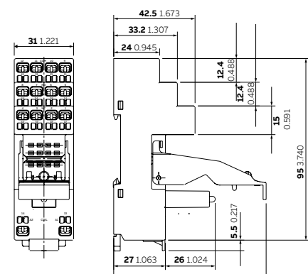
CR-M4LC - conexión por resorte
