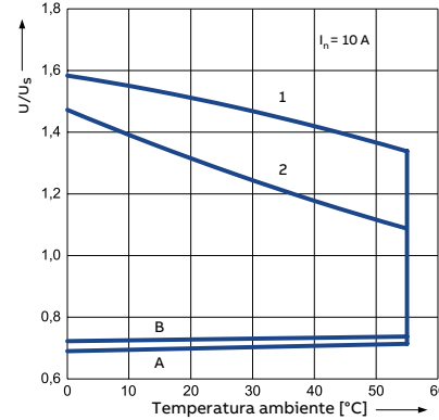
Alcance de la bobina de CA - 3 c/o
