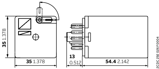
Relé CR-U con 3 contactos c/o
