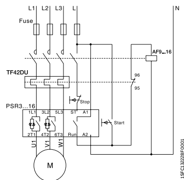
Con fusibles, contactor y sobrecarga
