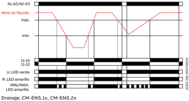
Drenaje: CM-ENS.1x, CM-ENS.2x
