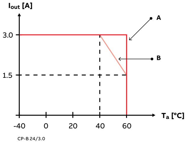
Curva característica de la temperatura con carga nominal
