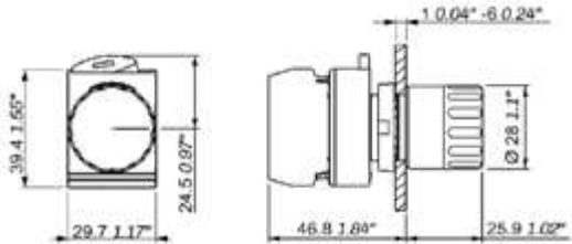
P9MPS Dimensiones (mm, pulgadas)
