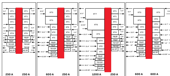
Caja central de 30" 40" offset box 45" offset box Caja central de 45"
