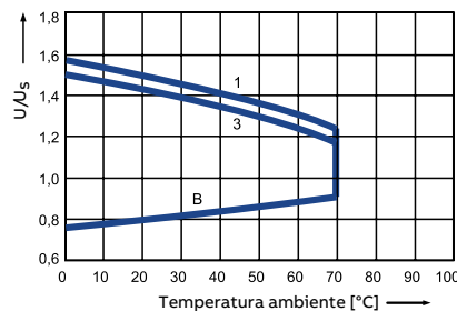
Alcance de la bobina de CA
