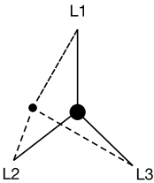
Desplazamiento del punto estrella
