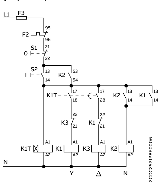
Esquema del circuito de control
