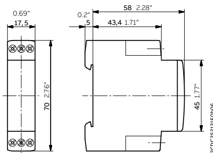
Dispositivos CT-D con 1 contacto c/o o 2 contactos n/o
