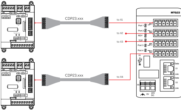
UMC100.3, aplicación montada fija con solución MTQ22-FBP.0/PNQ22-FBP.0
