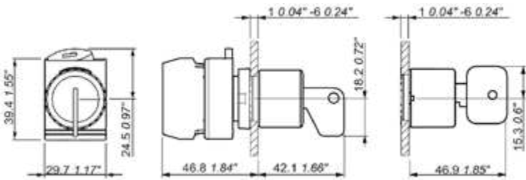
P9MSC..01, P9MSC..95
