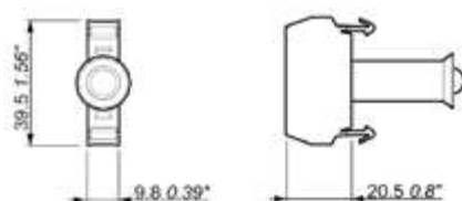
P9PL Dimensiones (mm, pulgadas)
