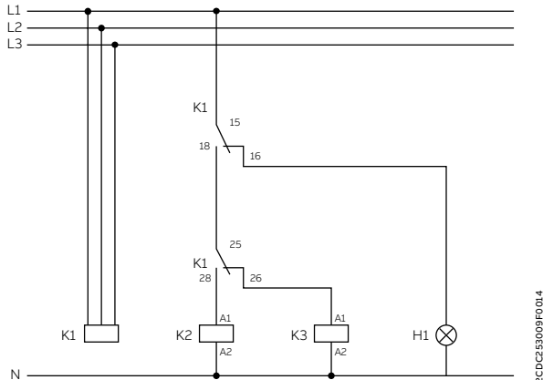
Esquema del circuito de control (K1 = CM-MPS.43 or CM-MPN.xx)
