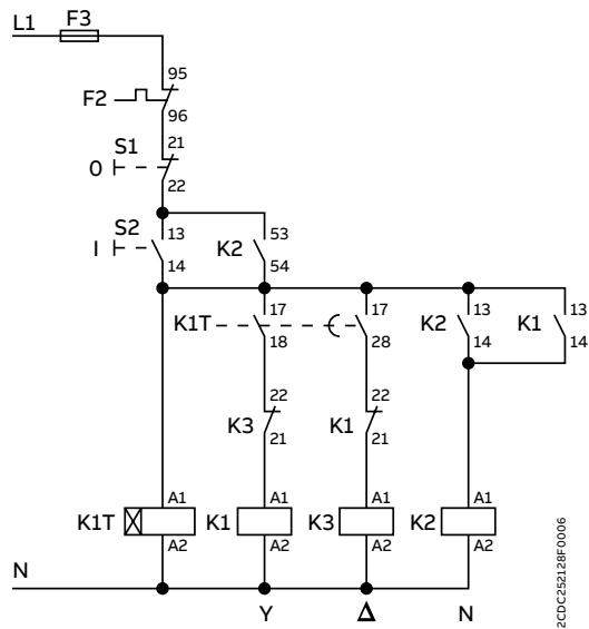
Esquema del circuito de control
