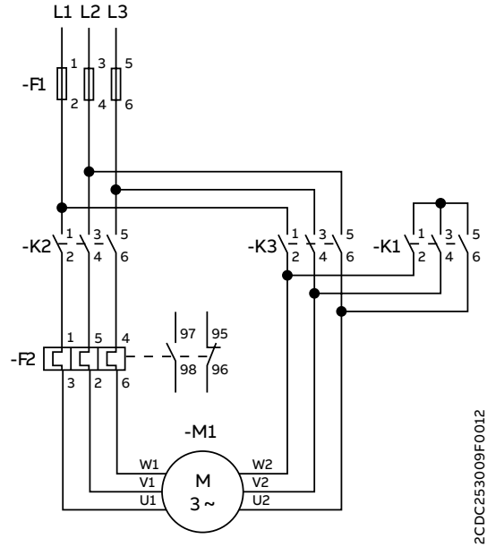
Circuito de potencia
