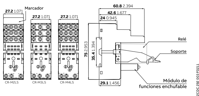
CR-M2LS(H) - CR-M3LS(H) - CR-M4LS - conexión por tornillo
