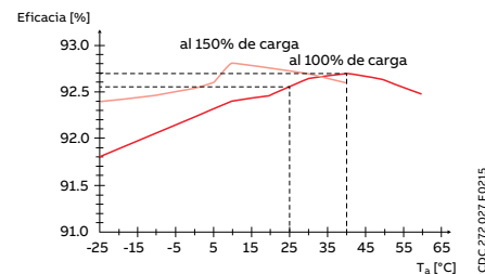
Rendimiento típico a temperatura ambiente
