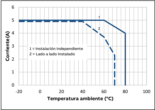
Salida MOS-FET CR-P
