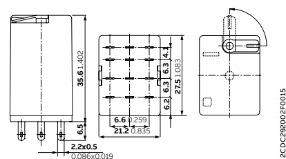
Relé CR-M con 3 contactos c/o
