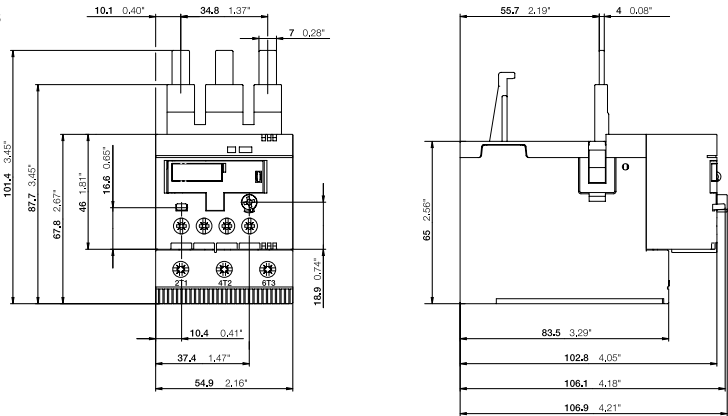
TF65
