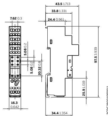
CR-PLC - conexión por resorte
