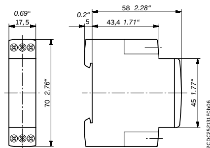
Dispositivos CT-C con 1 contacto c/o o 2 contactos n/o
