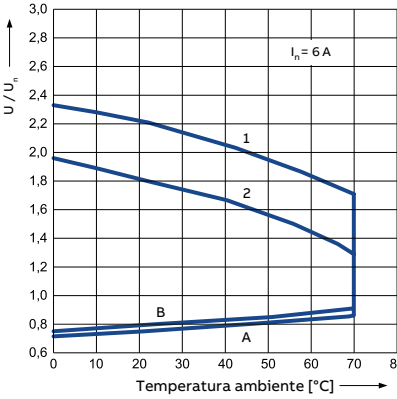
Alcance de la bobina de CC - 4 c/o
