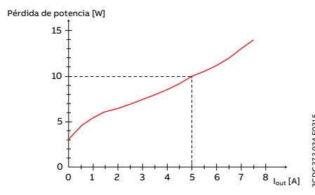
Pérdida de potencia típica en la corriente de salida
