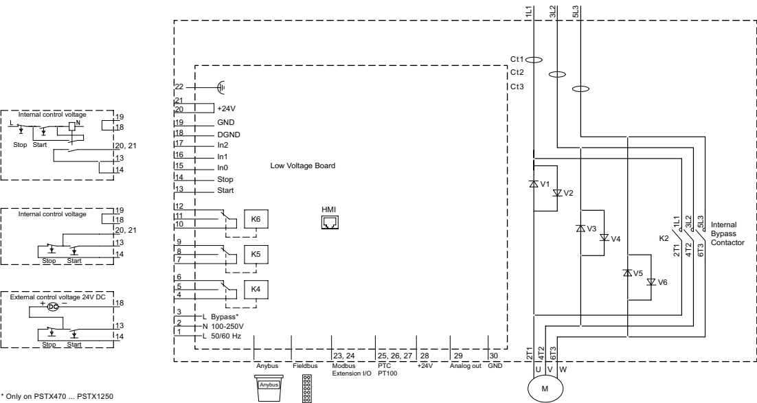
PSTX30 ... PSTX1250 Diagramas de circuitos de PSTX1250 según IEC
