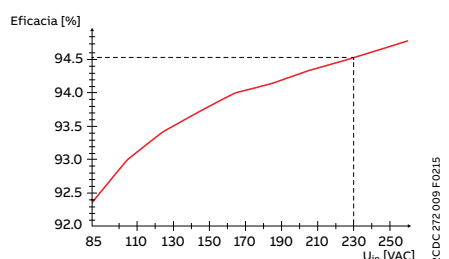
Eficiencia típica sobre la tensión de entrada de CA
