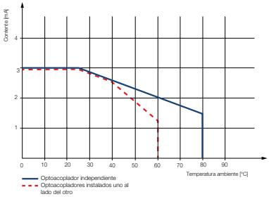
Curva de atenuación salida MOS-FET CR-S
