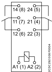
CR-P con 2 contactos c/o
