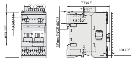
AF09Z..K, AF12Z..K, AF16Z..K Dimensiones principales mm, pulgadas
