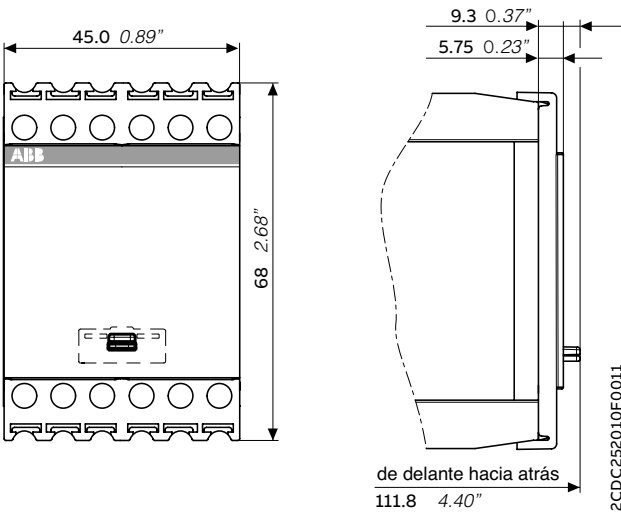
Tapa precintable COV:12
