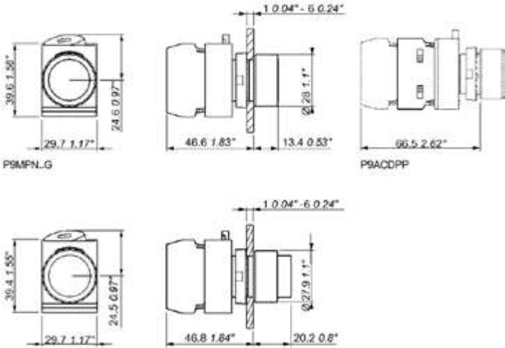
P9MPNLS Dimensiones (mm, pulgadas)
