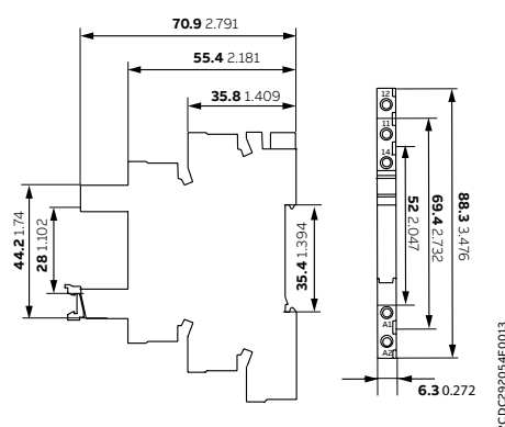
Enchufe CR-S - conexión por tornillo
