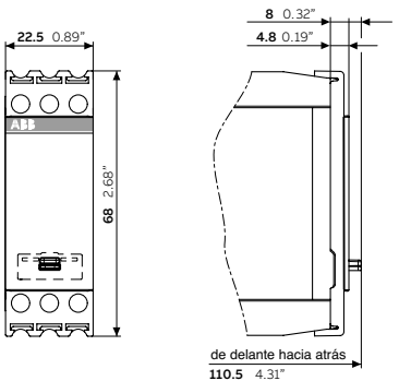
COV.11 tapa transparente precintable
