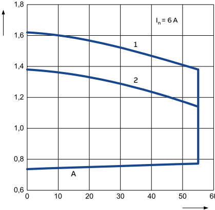
Alcance de la bobina de CA - 4 c/o
