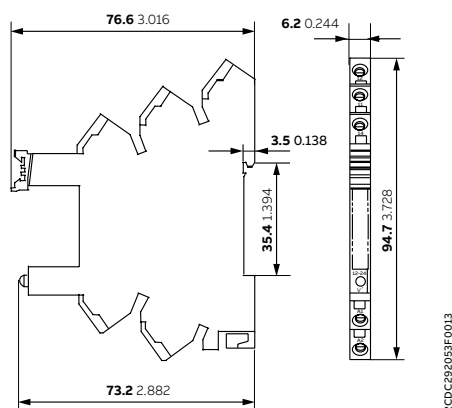
Enchufe CR-S - conexión por resort
