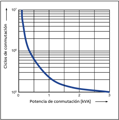
CR-M con 2 contactos c/o
