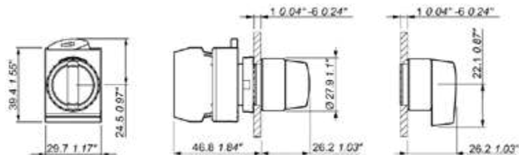
P9MSL, P9MSA
