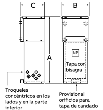
Dimensiones Fase única
