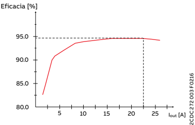
Eficiencia típica sobre la corriente de salida
