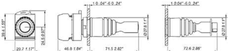
P9MMN, P9MMB Dimensiones (mm, pulgadas)
