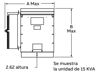
Dimensiones Tres fases
