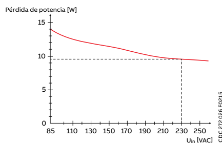
Pérdida de potencia típica sobre la tensión de entrada de CA
