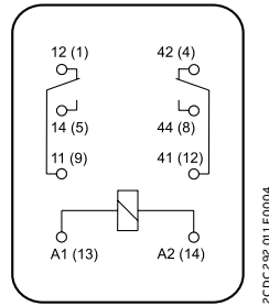
CR-M con 2 contactos c/o
