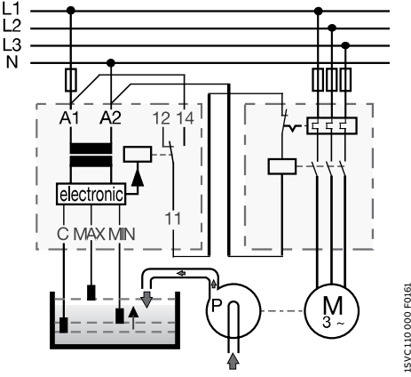
Control del nivel de líquido - llenado - función seleccionada "↑" (UP)
