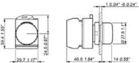
P9ML...D Dimensiones (mm, pulgadas)
