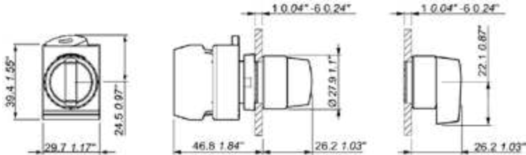
P9MSM, P9MSV Dimensiones (mm, pulgadas)
