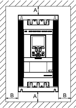
Distancia mínima a la pared
