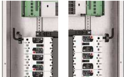
Ilustración de CT de núcleo dividido BCM, abierto y cerrado
