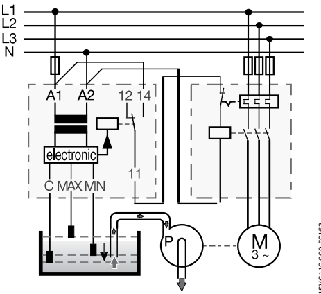
Control del nivel de líquido - vaciado - función seleccionada "↓" (Abajo)
