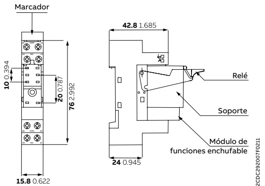
CR-PSS - conexión por tornillo
