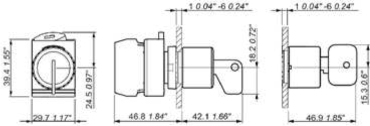
P9MSC..01, P9MSC..95 P9MSC..37 Dimensiones (mm, pulgadas)
