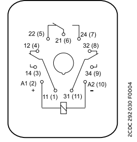
CR-U con 3 contactos c/o
