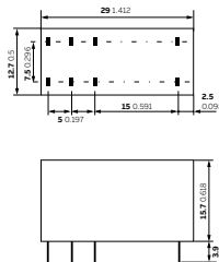
Relé CR-P
