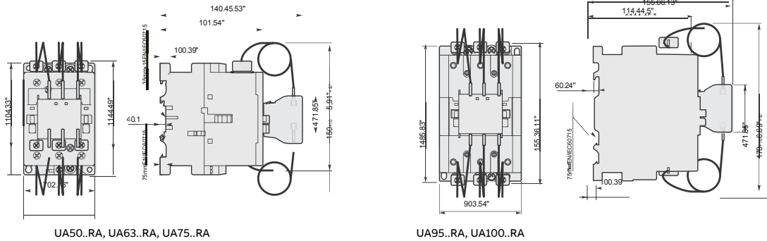
Dimensiones principales mm, pulgadas
