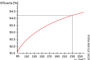
Eficacia típica sobre la tensión de entrada de CA
