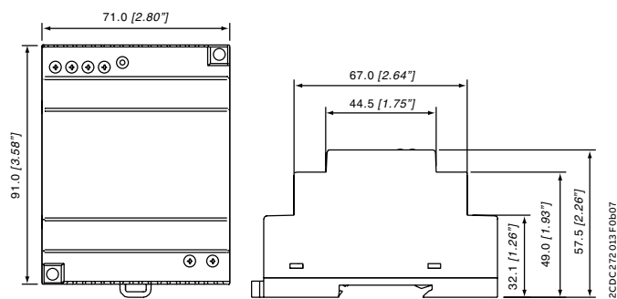
CP-D 24/2.5
