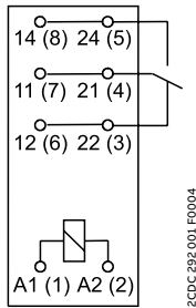
CR-P con 1 contacto c/o
