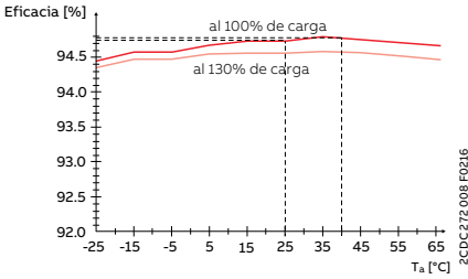
Rendimiento típico a temperatura ambiente
