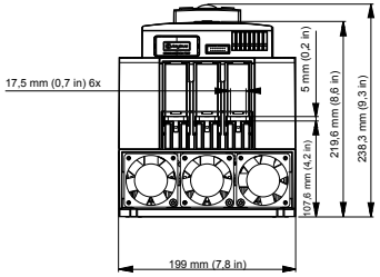
PSTX142 ... PSTX170
