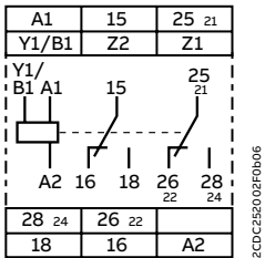
CT-MVS.21
