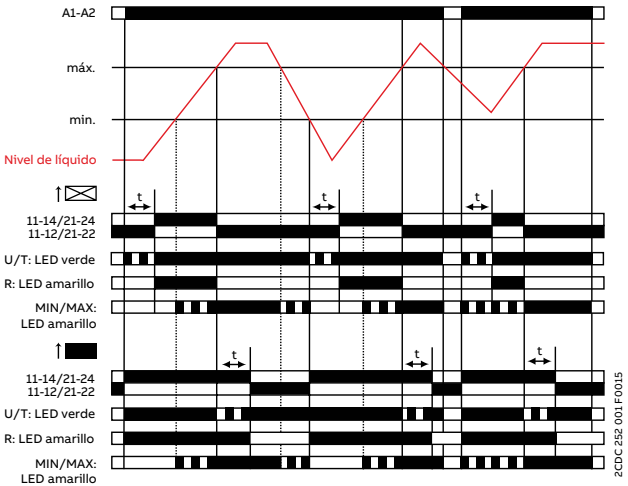
Relleno: CM-ENS.31
