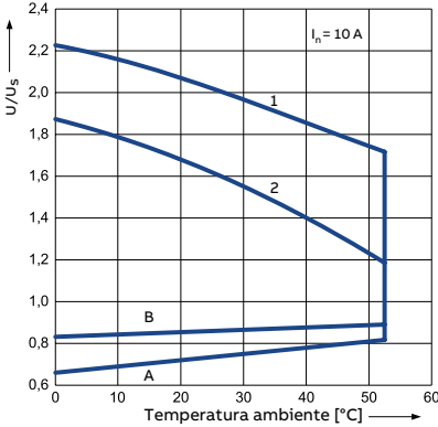
Alcance de la bobina de CC - 3 c/o
