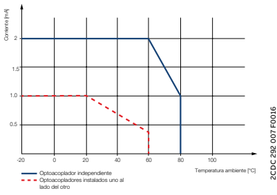
Curva de reducción de potencia salida triac CR-S
