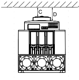
Distancia mínima al frontal
