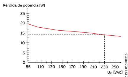
Pérdida de potencia típica sobre la tensión de entrada de CA
