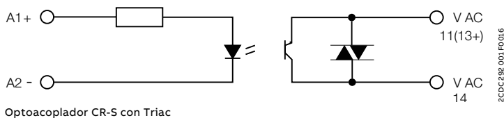
Optoacoplador CR-S con Triac
