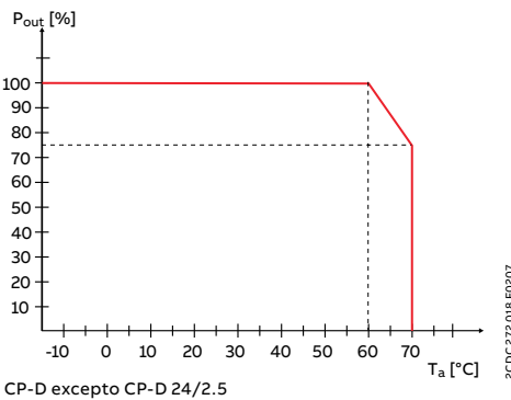
Curva característica de temperatura a tensión nominal de salida
