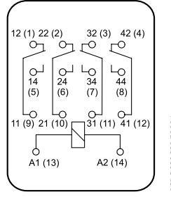
CR-M con 4 contactos c/o
