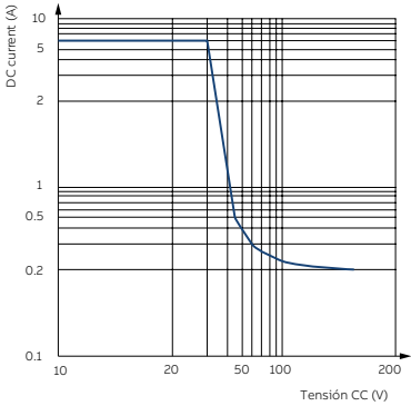
Máx. Capacidad de ruptura con carga CC
