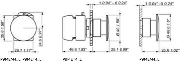
Dimensiones (mm, pulgadas)
