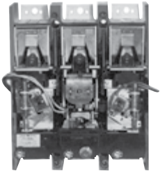
Interruptor automático de bastidor en J con accesorios internos montados en cada polo
