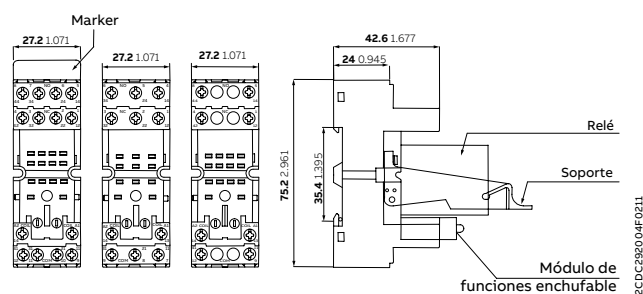
CR-M2SS - CR-M3SS - CR-M4SS - conexión por tornillo
