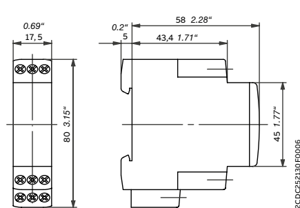
Dispositivos CT-C con 2 contactos c/o
