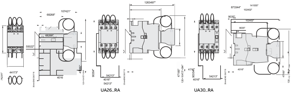
UA16..RA Dimensiones principales mm, pulgadas
