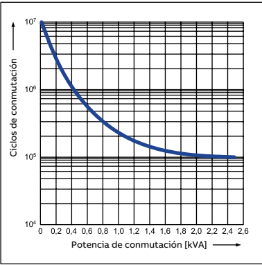
CR-M con 3 contactos c/o
