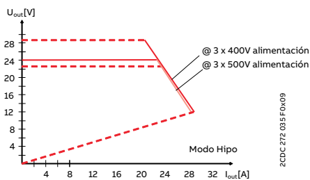
CP-T 24/20.0 Modo Hipo
