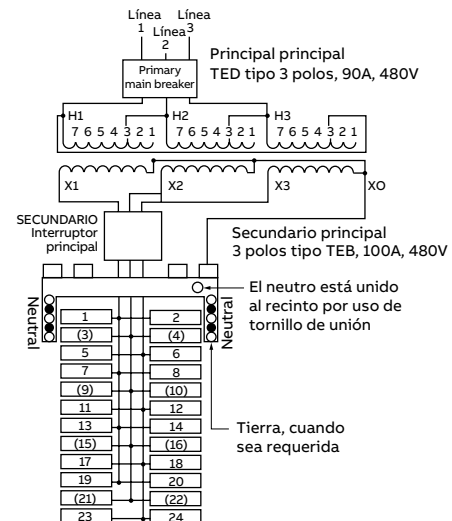
Diagrama de cableado trifásico 1
