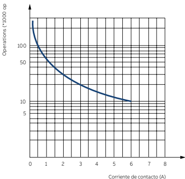
Curva de resistencia
