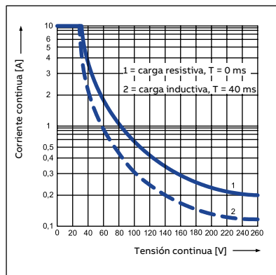
CR-M con 3 contactos c/o
