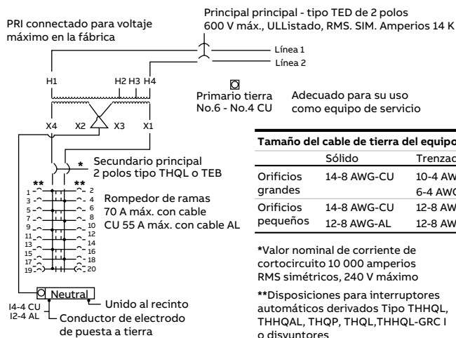
Diagrama de cableado típico Monofásico
