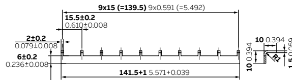
Barra de puentes CR-PJ
