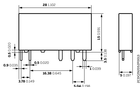
Relé CR-S
