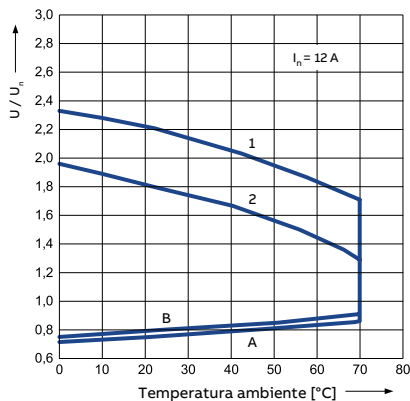
Alcance de la bobina de CC - 2 c/o
