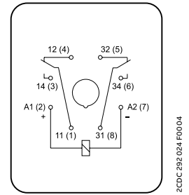
CR-U con 2 contactos c/o
