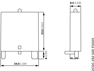
Módulo de funciones CR-Uxx
