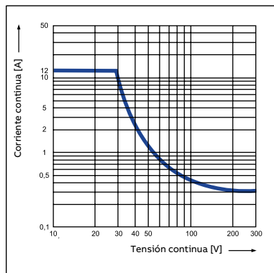
CR-M con 2 contactos c/o
