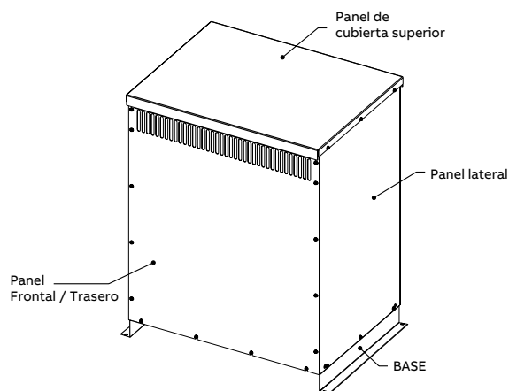
KIT CAJA: 1 TAPA + 2 LADOS + 2 FRENTE
