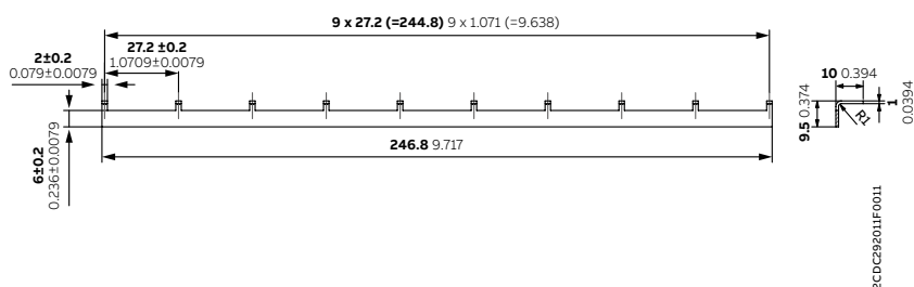
CR-MJ barra de puente
