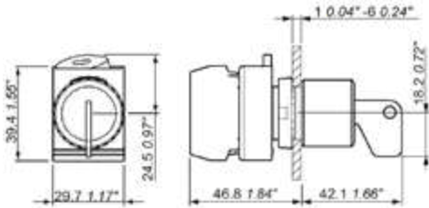
P9MSC..01, P9MSC..95 Dimensiones (mm, pulgadas)
