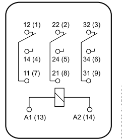
CR-M con 3 contactos c/o
