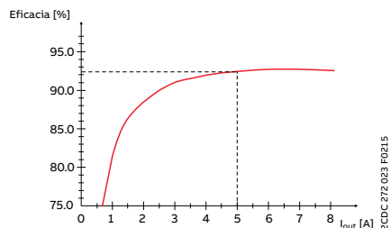
Eficiencia típica sobre la corriente de salida
