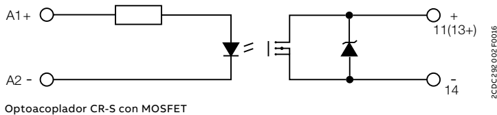
Optoacoplador CR-S con MOSFET
