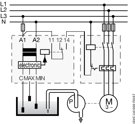
Control de nivel de líquido - drenaje
