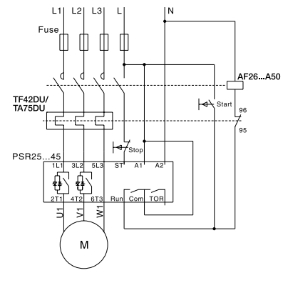
Con fusibles, contactor y sobrecarga
