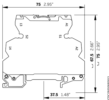
R600 - conexión por resorte
