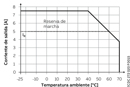
Curva característica de temperatura a U_{out} = 24\text{ V}
