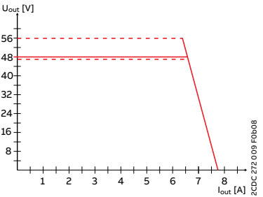
CP-E 48/5.0
