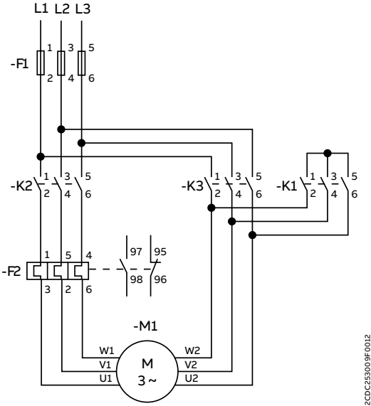
Circuito de potencia
