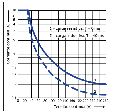
CR-U con 2 y 3 contactos c/o
