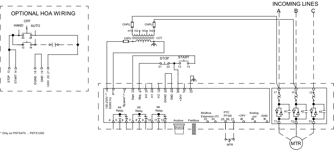
Diagramas de circuitos según UL
