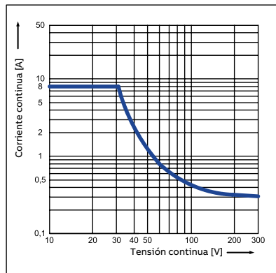
CR-P con 2 contactos c/o
