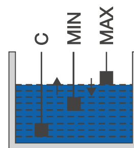
Modo de funcionamiento con tres electrodos
