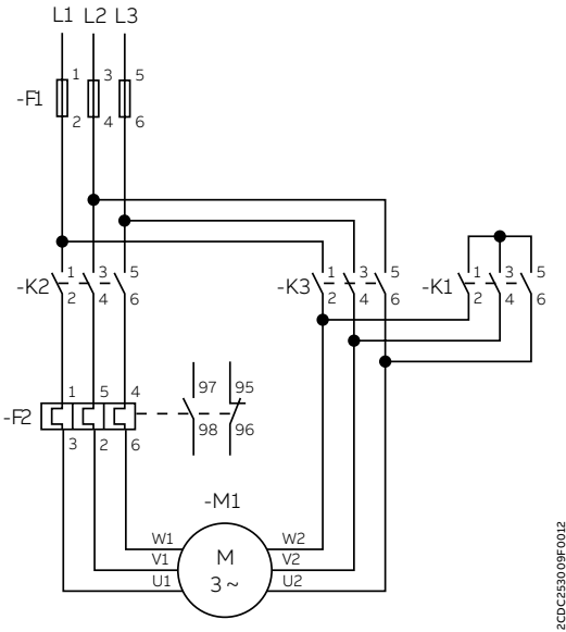
Esquema del circuito de control
