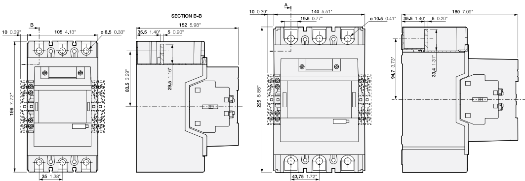
Dimensiones principales mm, pulgadas
