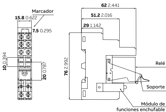
CR-PLS - conexión por tornillo
