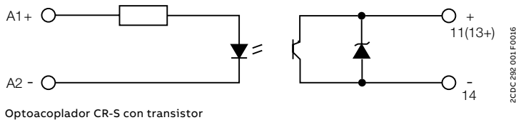
Optoacoplador CR-S con transistor
