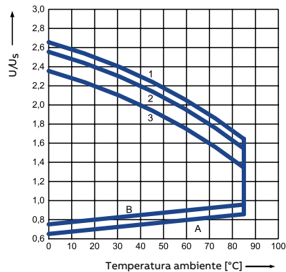
Campo de funcionamiento de la bobina de CC
