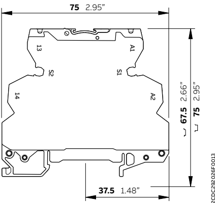
R600 - conexión por resorte
