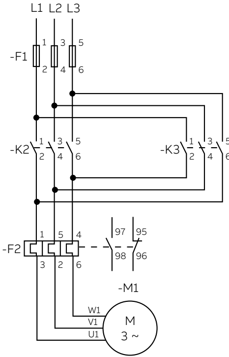
Esquema del circuito de potencia
