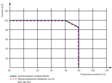
Curva de reducción de potencia Salida transistor CR-S
