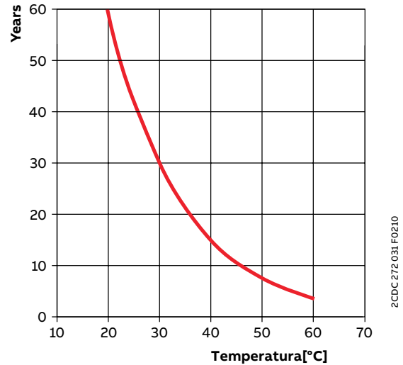
Vida útil de los condensadores en función de la temperatura
