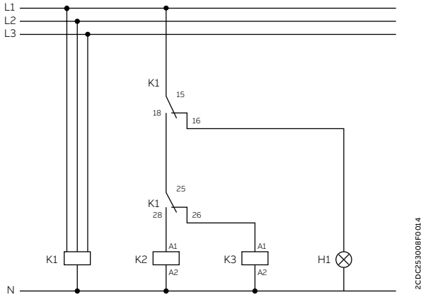
Esquema del circuito de control (K1 = CMMP5.23)
