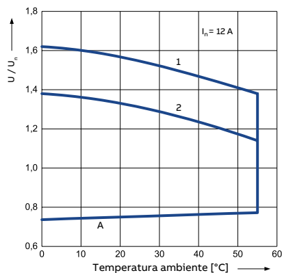
Alcance de la bobina de CA - 2 c/o
