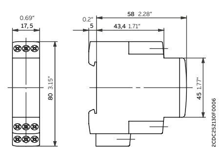
Dispositivos CT-D con 2 contactos c/o
