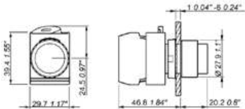
P9MPN..S Dimensiones (mm, pulgadas)
