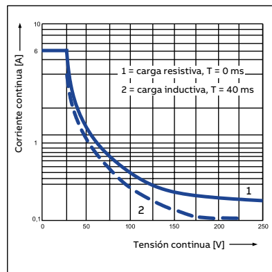
CR-M con 4 contactos c/o
