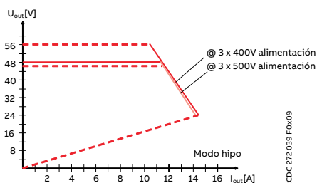
CP-T 48/10.0 Modo hipo
