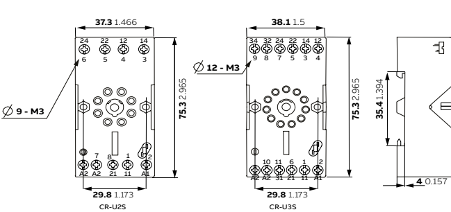
CR-U2S - CR-U3S - conexión roscada
