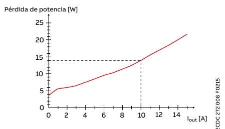
Pérdida de potencia típica en la corriente de salida
