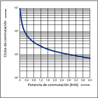
CR-P con 1 contacto c/o
