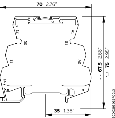
R600 - conexión por tornillo
