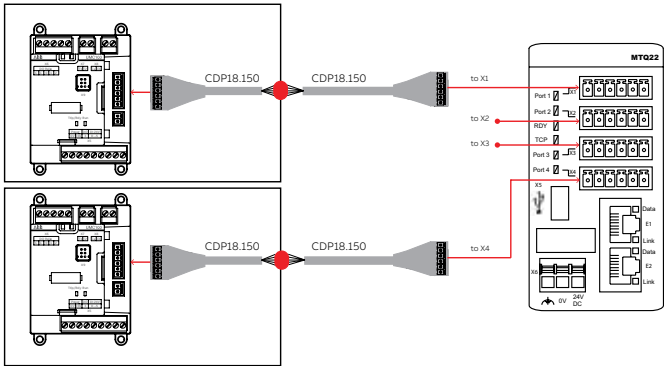
UMC100.3, solicitud retirable con MTQ22-FBP.0/PNQ22-FBP.0
