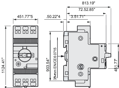
MS132-K > 10A Dimensiones principales mm, pulgadas
