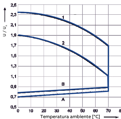
Alcance de la bobina de CC - 3 c/o
