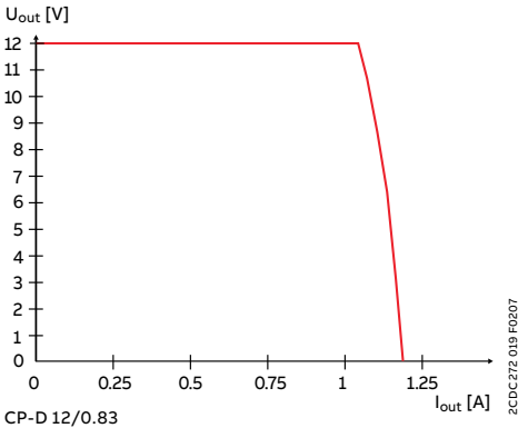
Curva característica de salida a T_a = 25\text{ °C}
