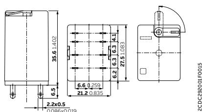
Relé CR-M con 2 contactos c/o
