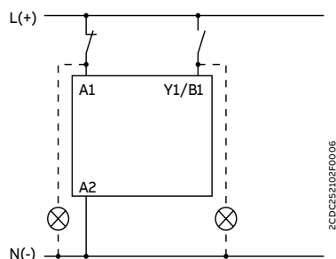
Dispositivos CT-C con 1 contacto c/o o 2 contactos n/o
