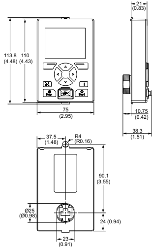
Teclado desmontable del PSTX
