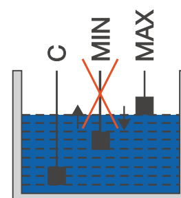
Modo de funcionamiento con dos electrodos
