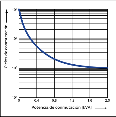
CR-P con 2 contactos c/o
