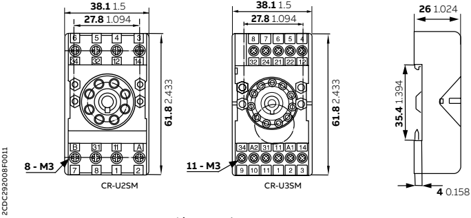
CR-U2SM - CR-U3SM - conexión roscada
