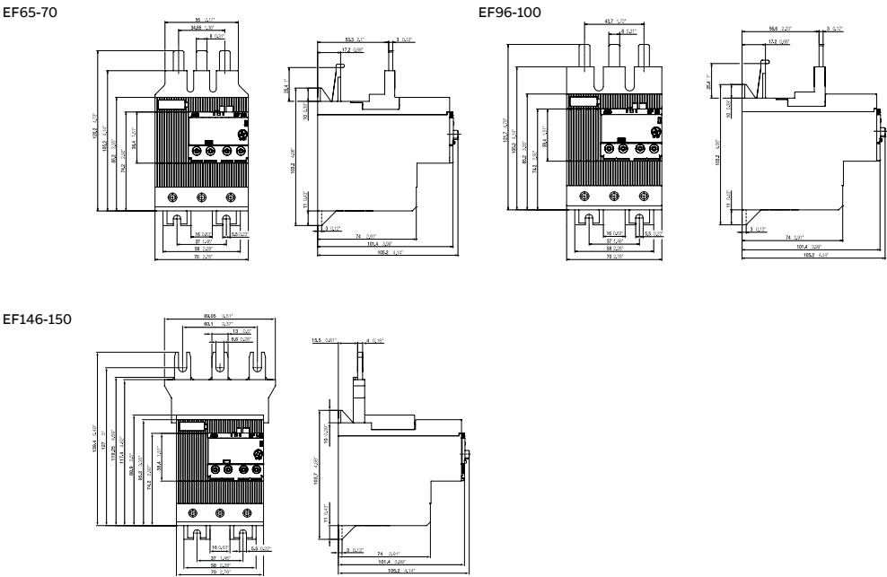
Dimensiones principales mm, pulgadas
