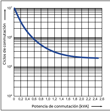
CR-U con 2 y 3 contactos c/o
