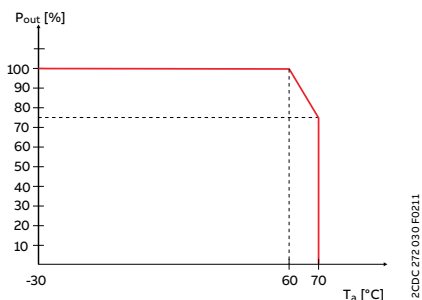
CP-T 24/20.0, CP-T 48/10.0
