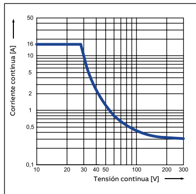
CR-P con 1 contacto c/o
