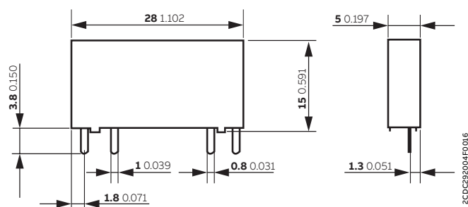
Optoacoplador CR-S
