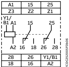
CT-MXS.22
