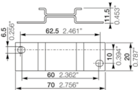
Adaptador ADP.01 para montaje con tornillos
