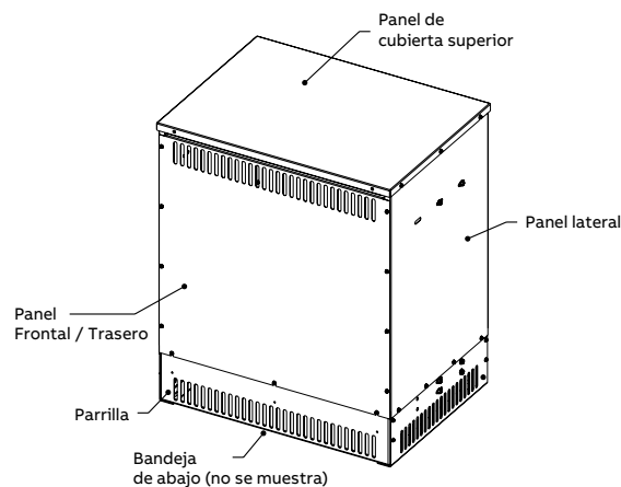
KIT CAJA: 1 TAPA + 2 LADOS + 2 FRENTE
