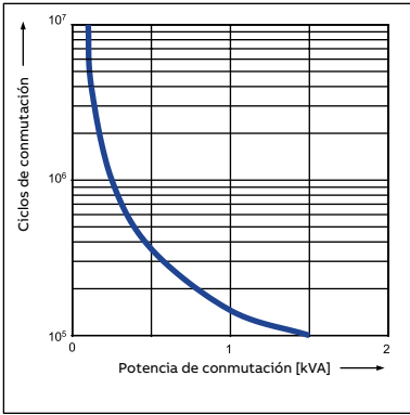
CR-M con 4 contactos c/o
