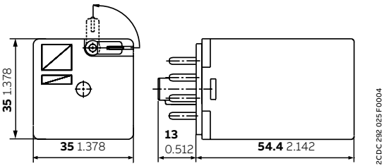
Relé CR-U con 2 contactos c/o
