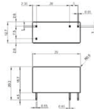
Optoacoplador CR-P
