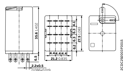
Relé CR-M con 4 contactos c/o
