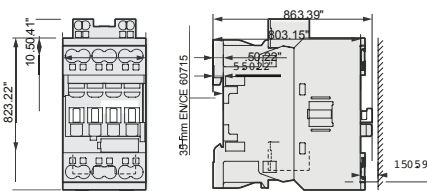
AF26Z..K, AF30Z..K, AF38Z..K
