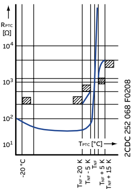
Características del sensor de temperatura
