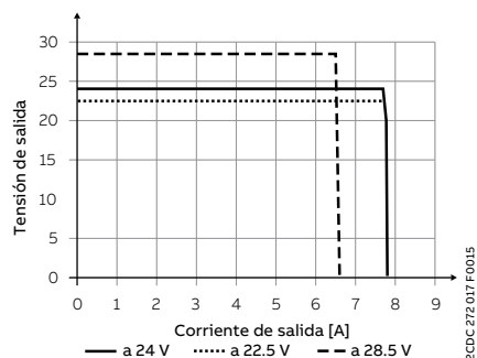
Curva característica de salida a T_a = 25^\circ\text{C}
