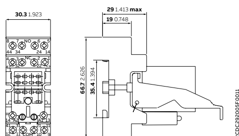
CR-MxSF - conexión por tornillo
